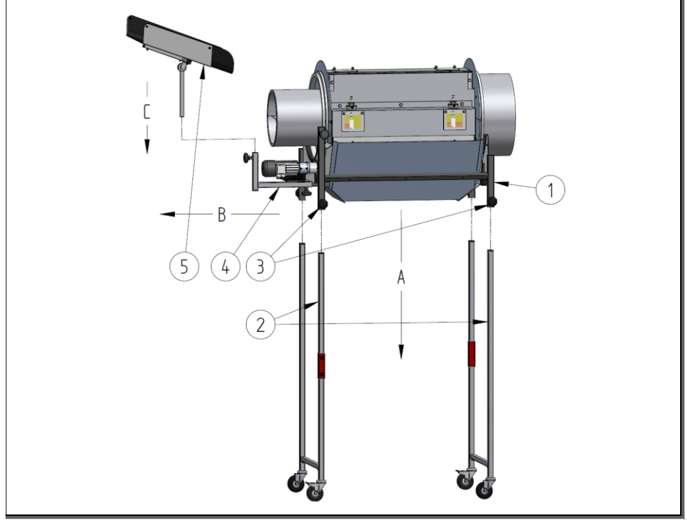
Şekil 8: Montaj
