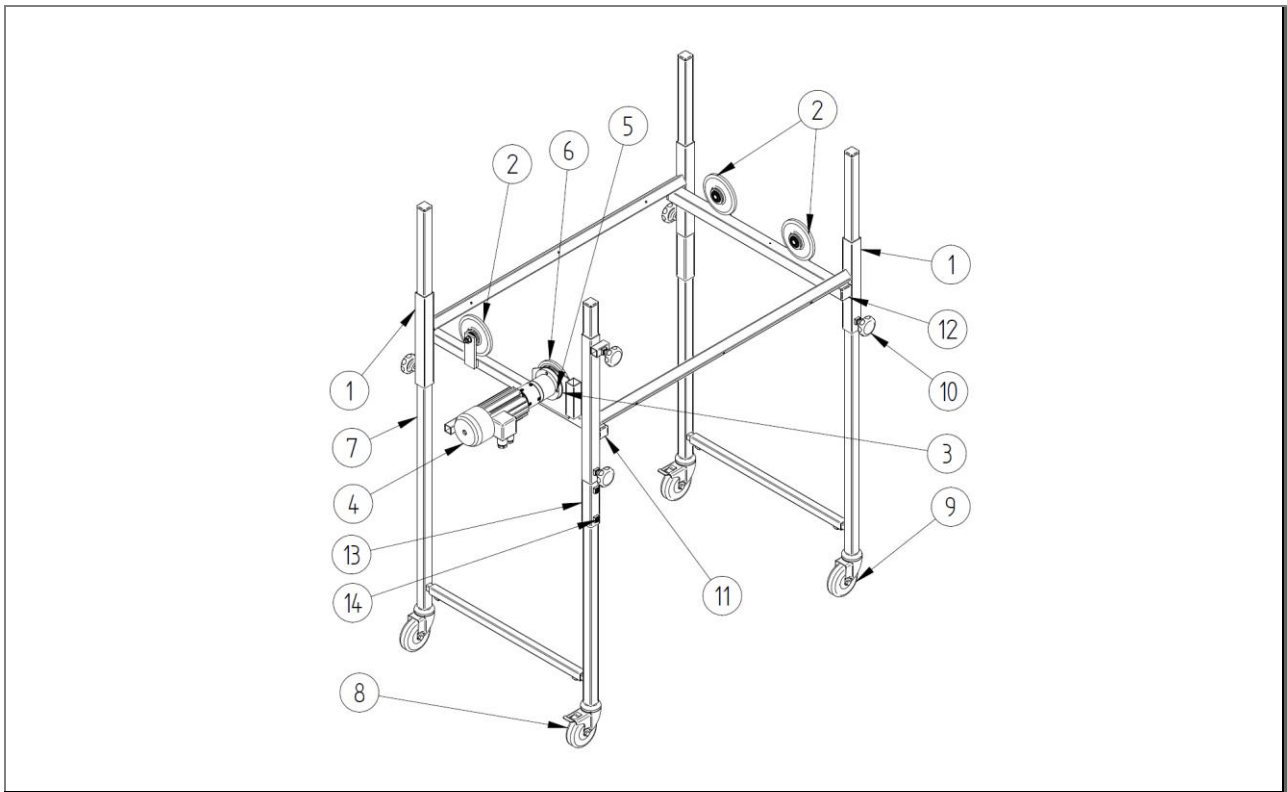
Obr. 19: Kusovník: Spodní rám - separační buben - ZZ.860.0003
